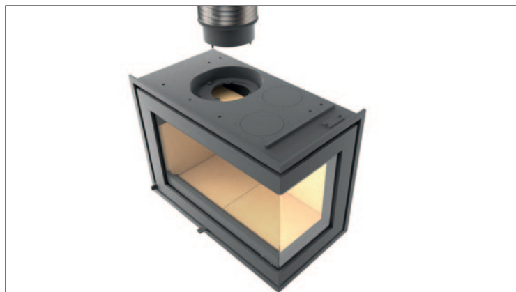
Axe de la sortie de fumée ajustable.
